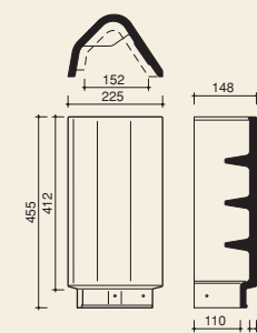
Pultfirstziegel (2,5 Stück/m)
