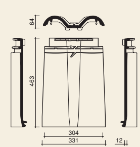
Doppelwulstziegel
