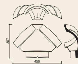
Walmkappe (dreiachsig)
