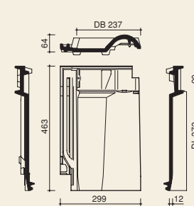
Firstanschlussziegel
