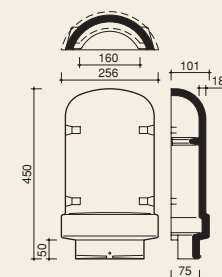
Grat-Anfangziegel
