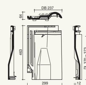
Lüfterziegel mit Gitter (LQ = 22,0 cm 2 )
