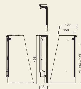
Ortgangsteg, rechts
